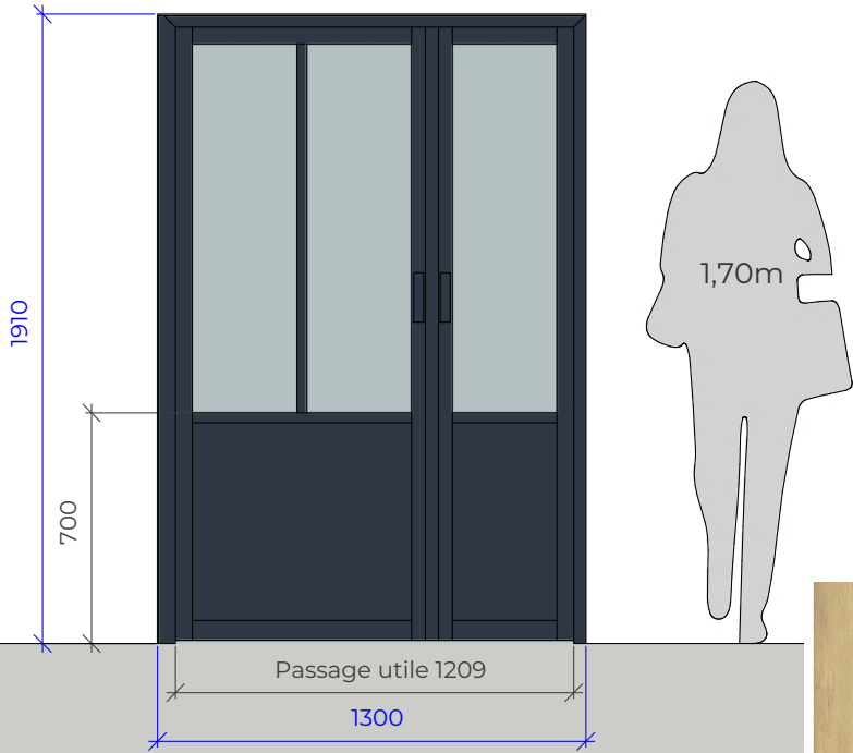
targette haute et basse sur vantail semi fixe
